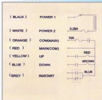
F21-2S接線圖
