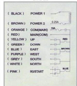
F21-E1/E1B接線圖
