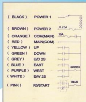
F21-4D接線圖
