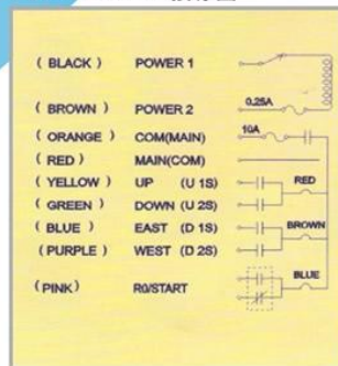
F21-4S/4SB/2D接線圖
